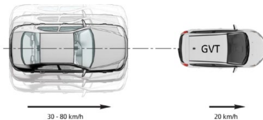
圖 7b：前車移動情境試驗
