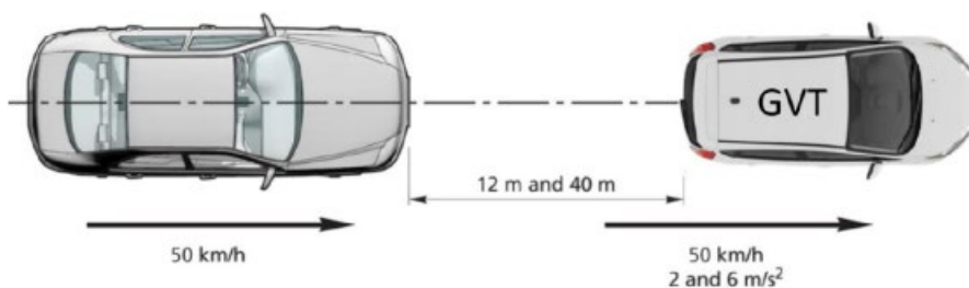
圖 7c：前車煞車情境試驗
