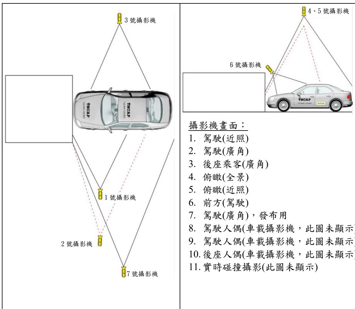
圖 4：攝影機 1 至 7 號位置(前方全寬撞擊剛性碰撞壁)
