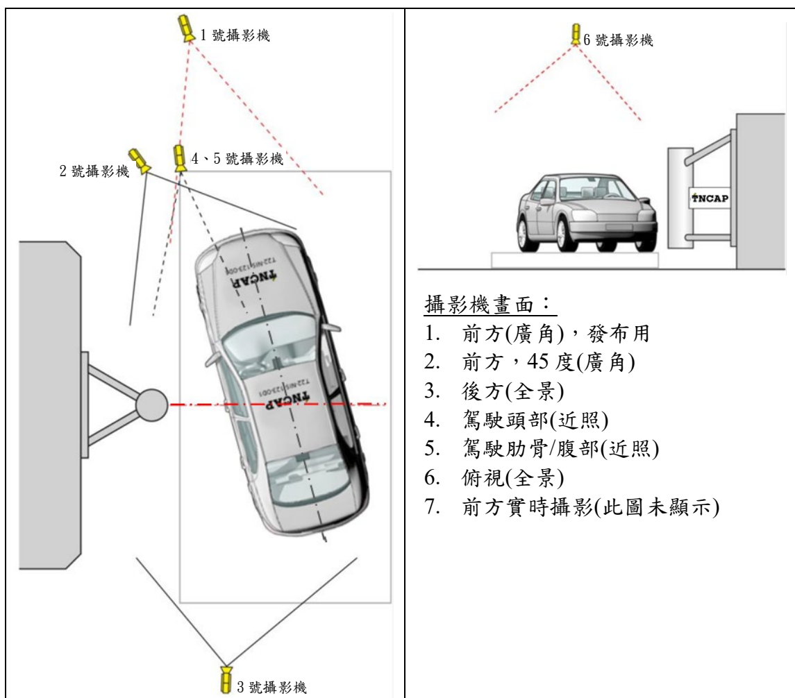
圖 6：攝影機 1 至 6 號位置(側方斜角立柱)
