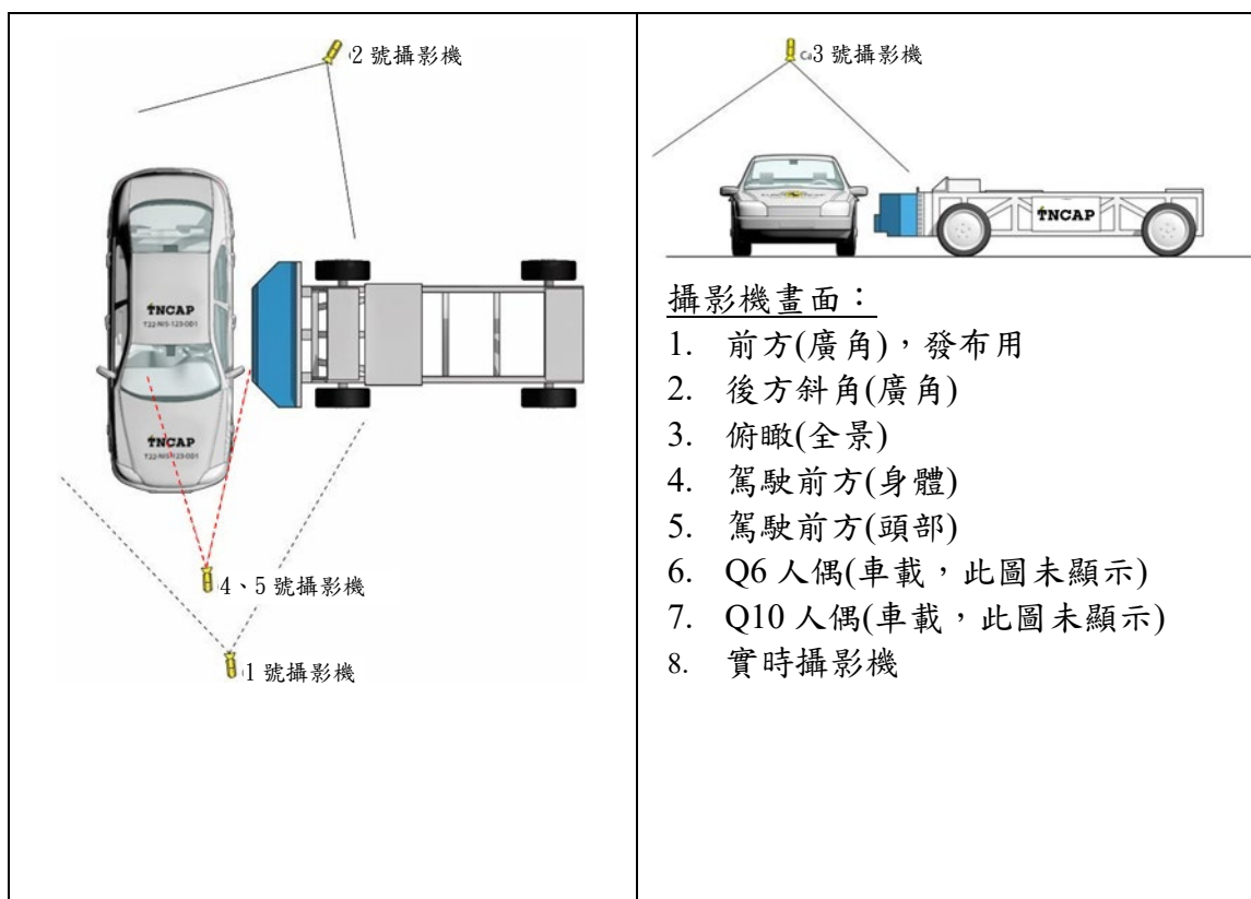
圖 5：攝影機 1 至 5 號位置(側方撞擊移動式可變形碰撞壁)
