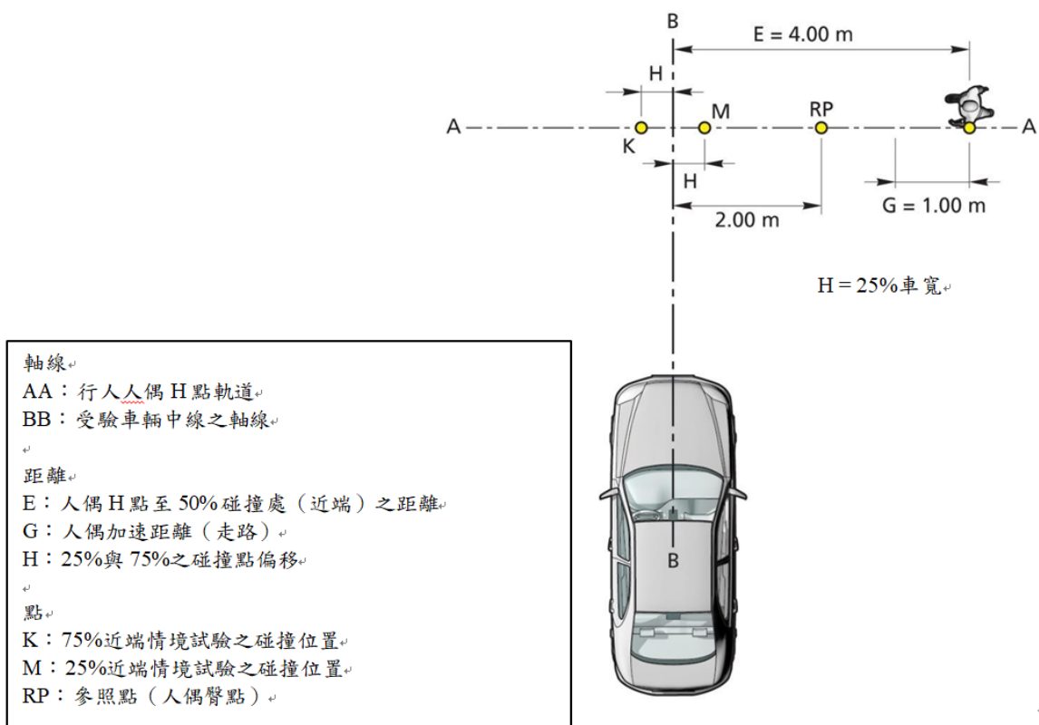
圖 8b：近端成人碰撞情境試驗 25% 及近端成人碰撞情境試驗 75%，成人行人自近端走路穿越其路徑
